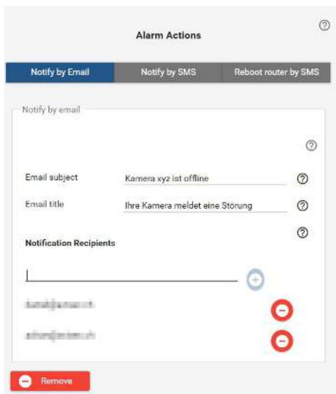
Abbildung 4: Empfänger für Alarmierung konfigurieren (avisec cloud)
